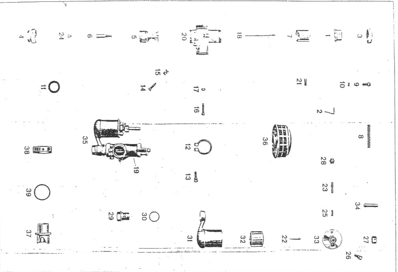
Tafel 19 Amdel-Vergaser Typ 76/424 (Sportmaschine)
